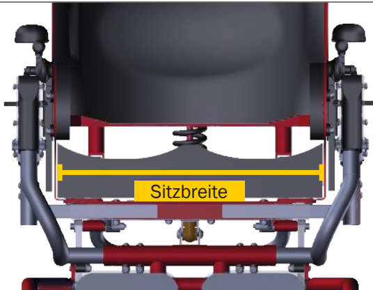
ERGO-Variante (Ansicht von vorne)
